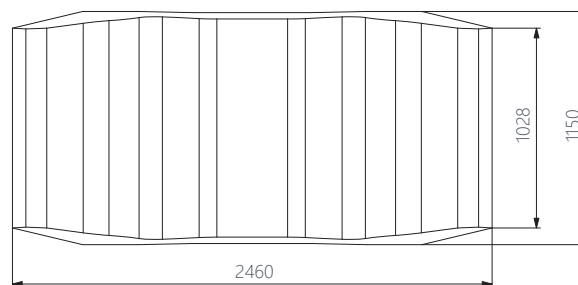
draufsicht & ansicht / top view & side view
