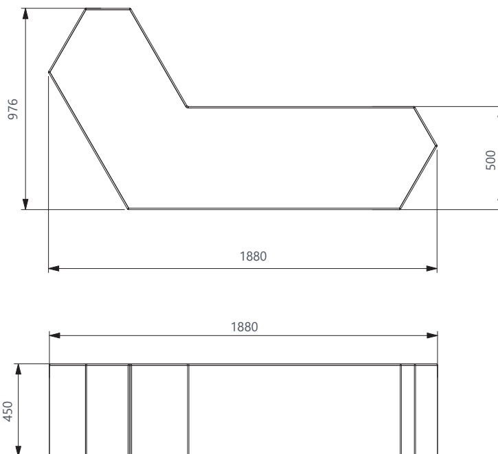
draufsicht & ansicht / top view & side view
