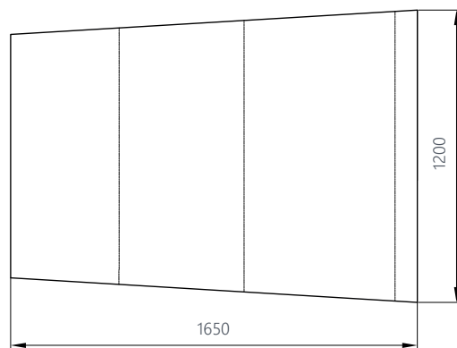
draufsicht & ansicht / top view & side view
