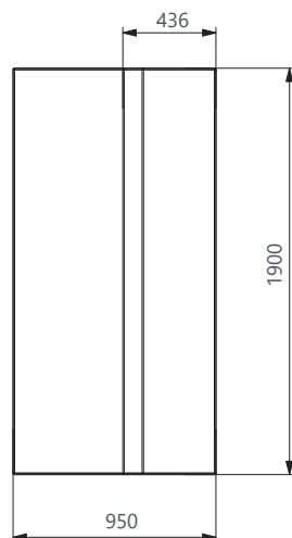
draufsicht & ansicht / top view & side view
