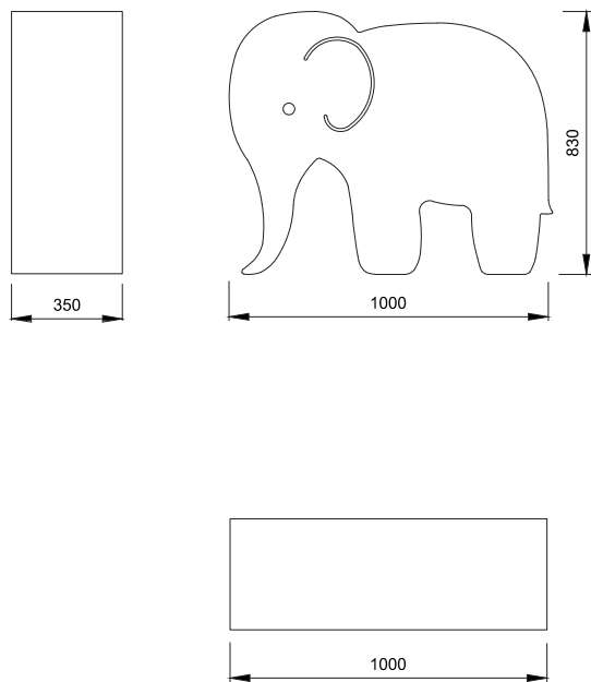
draufsicht & ansicht / top view & side view
